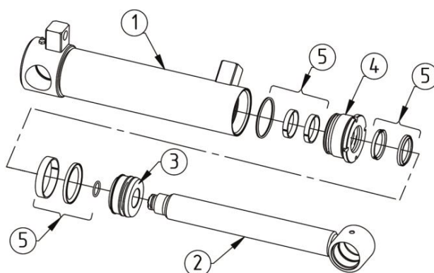
152.09.00.00.00 Гидроцилиндр грейфера
